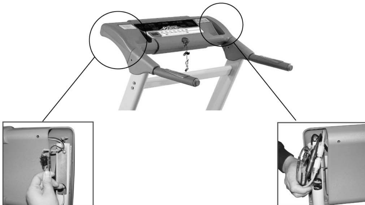
Rechts van vooraanzicht (sluit de 2 kabels aan als afgebeeld)
